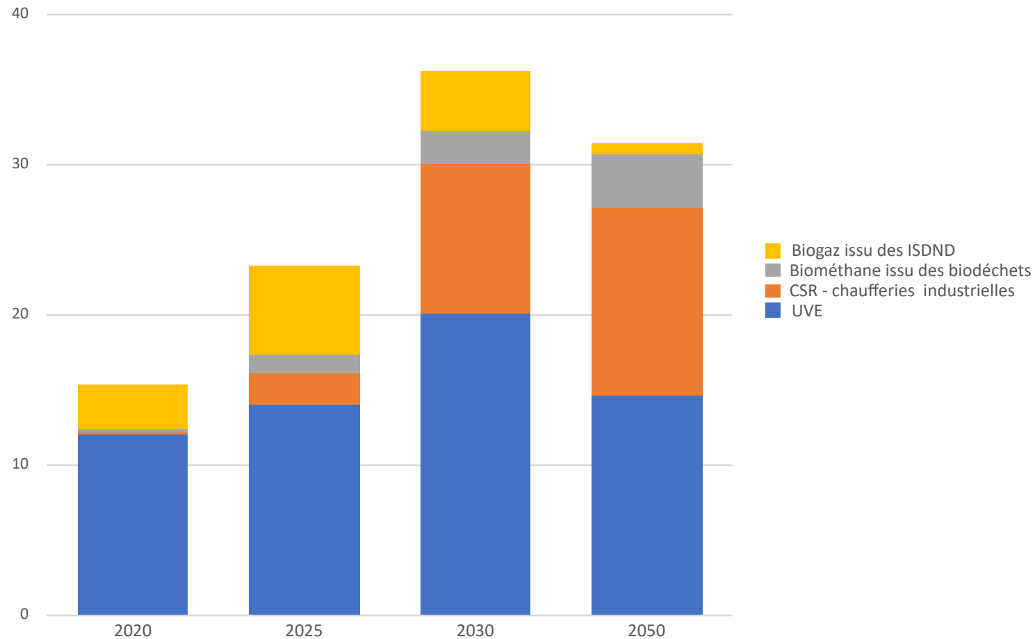
Evolution de la production d'énergie (biogaz ou chaleur) en TWh à partir des déchets à l'horizon 2050
